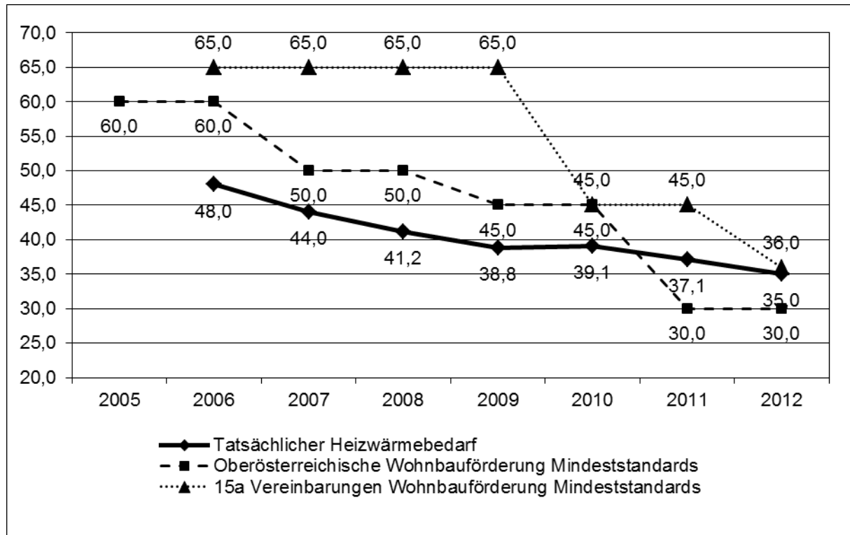
Abbildung 1: Vergleich von Heizwärmebedarf-Mindeststandards und tatsächlichem Heiz-wärmebedarf von Neubauten in Oberösterreich von 2005 bis 2012 (in kWh/m 2 ) 17
