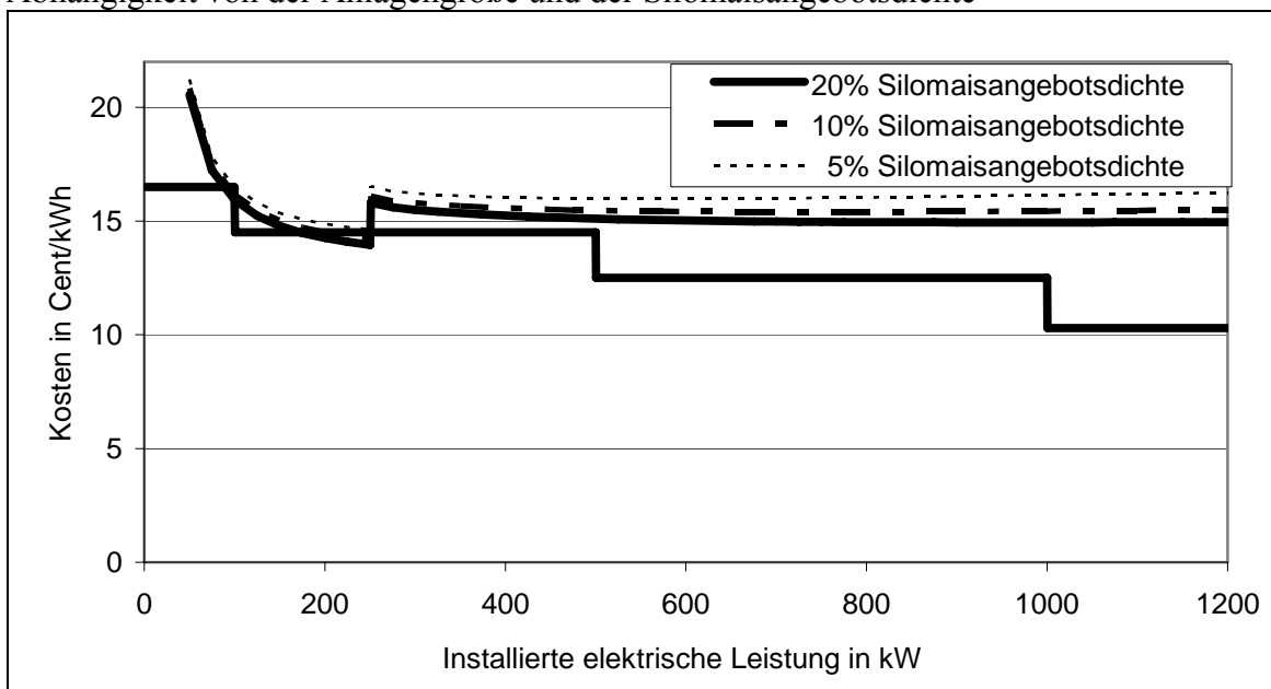
Ökostrompreis und Kosten je kWh unter Berücksichtigung der Investitionsförderung in Abhängigkeit von der Anlagengröße und der Silomaisangebotsdichte
