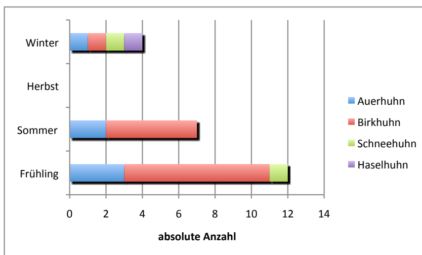
Abb. 32: Absolute Anzahl an Kollisionsopfern innerhalb der 4 Saisonen, aufgeteilt nach Raufußhuhnarten (n = 23)
