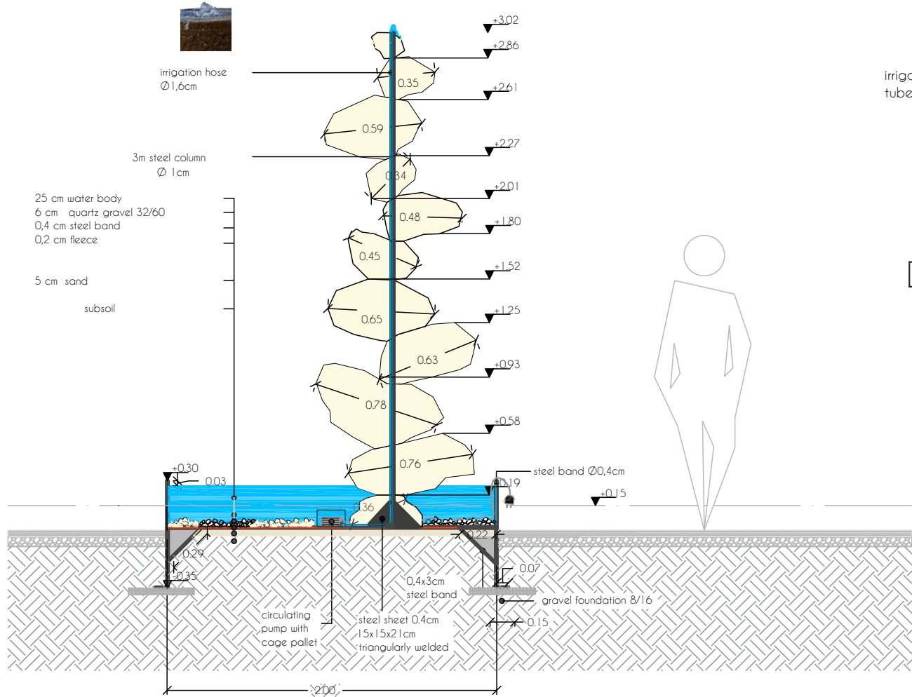
S3 M 1:25
