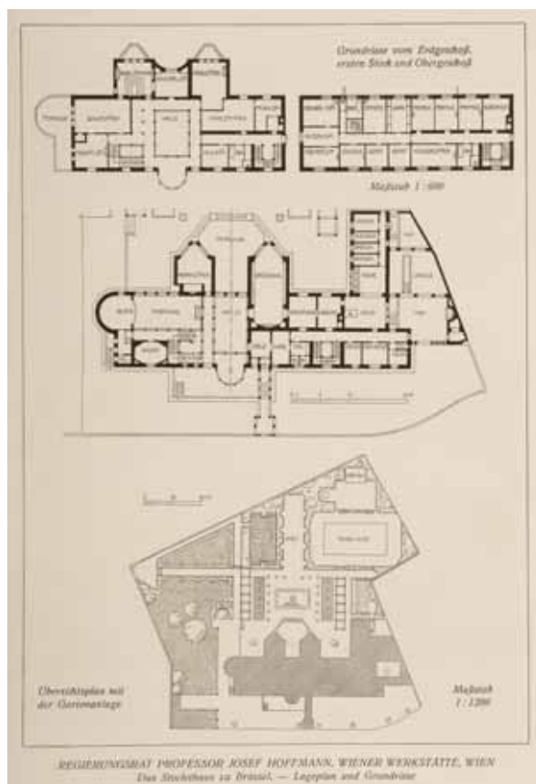
Grundrisse vom Haus, Übersichtsplan vom Garten Stoclet (die Pergolen sind falsch gezeichnet, sieben haben je 7 Kompartimente) (© MAK, Wien, aus: Moderne Bauformen I , 1914, S. 6)
