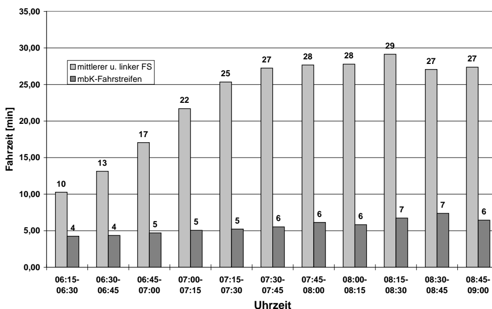
Abb. 2.6-1: Vergleich der mittleren Fahrzeiten der mbK-Fahrstreifen-Benutzer und der übrigen Kfz je Viertelstunde in Fahrtrichtung Linz auf der B127 von 6:15 bis 9:00 Uhr (Querschnitt X-Dorf, Montag 10.05.1999)
