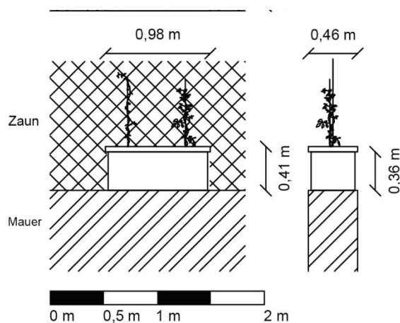
Abb. 27: Schematische Skizze eines Pflanztröges.
