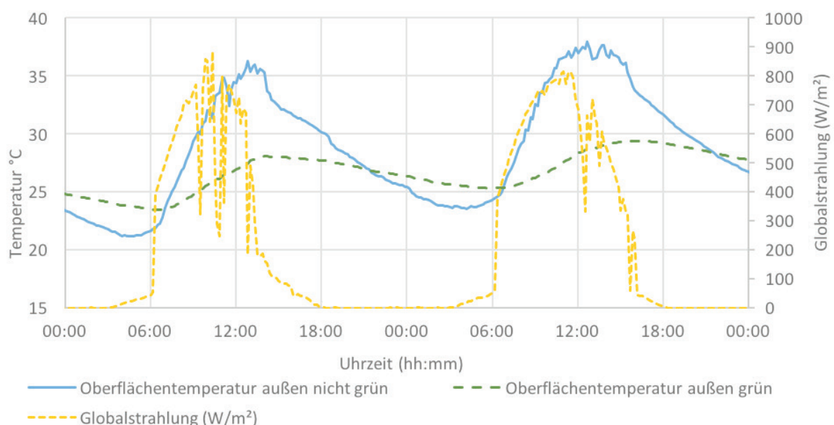
Abb. 56: Oberflächentemperatur der Fassade außen. Ohne Begrünung und mit Begrünung mittels Trogsystem.
