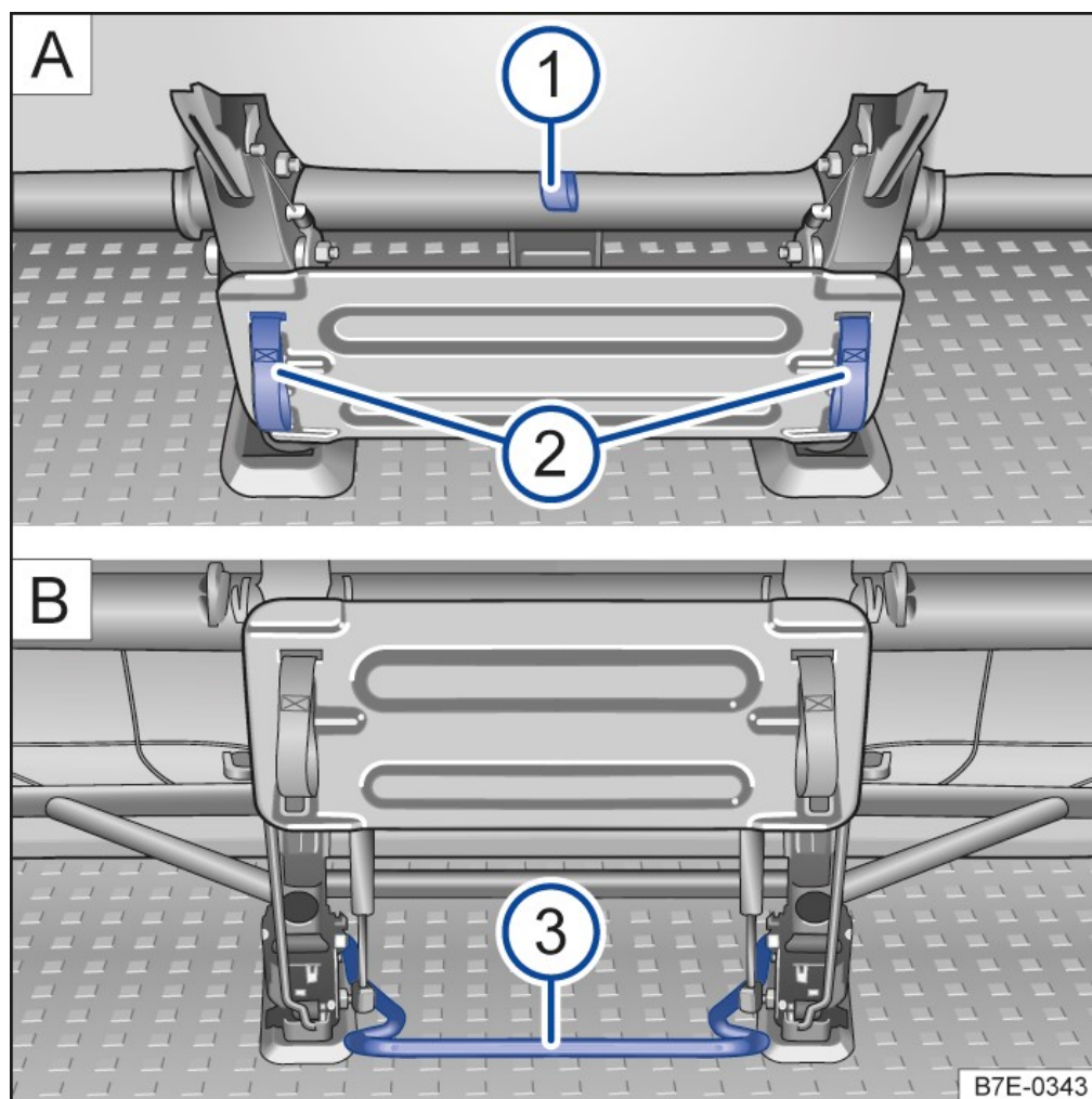
Abb. 1 An der Unterseite der Dreier-Sitzbank: Bedienelemente zum Klappen der Dreier-Sitzbank.
