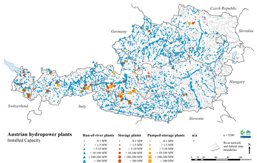
Abb. 2. Wasserkraftwerke in Österreich klassifiziert nach den Kraftwerkstypen Laufkraftwerk, Speicherkraftwerk und Pumpspeicherkraftwerk, Status: 2012 (Habersack et al., 2012; Wagner et al., 2015).
