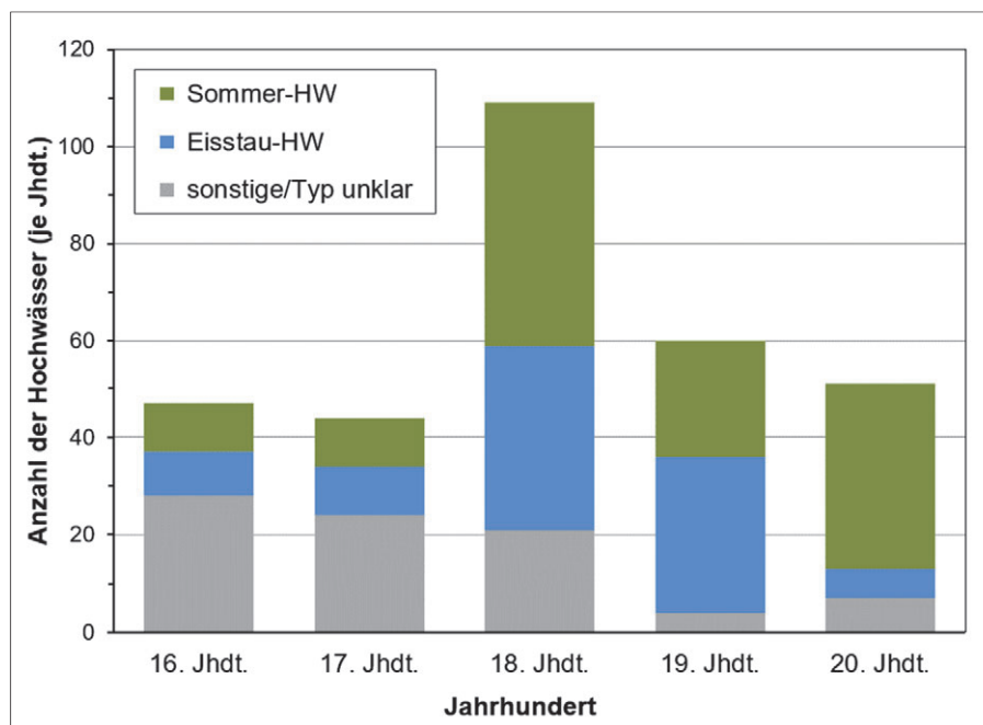
Abb. 5: Verteilung der historisch überlieferten Hochwasserursachen an der Wiener Donau seit dem 16. Jahrhundert.
