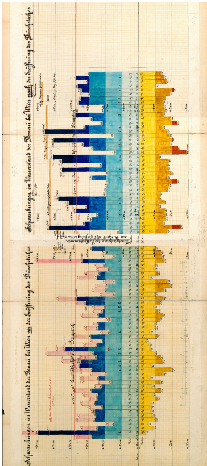
Abb. 4: Zunahme extremer Wasserstände an der Wiener Donau: vor der Regulierung 1829 – 1870 und nach der Regulierung 1875 – 1913 (siehe schwarze und rote Balken, rosa Balken beziehen sich auf den Donaukanal; WStLA 3.2.2.P23/1.119739.5).
