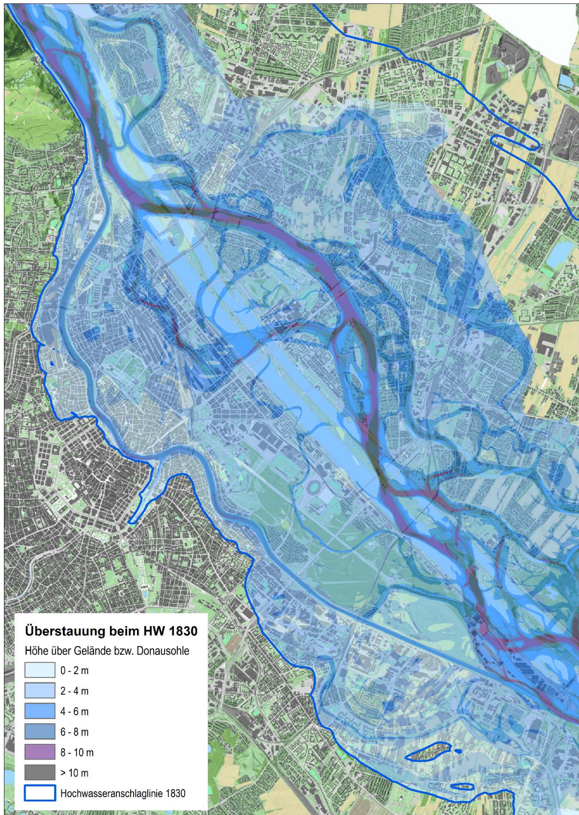
Abb. 6: Überschwemmungen in Wien beim Eisstoß-Hochwasser 1830. Die Überflutungen reichten im Marchfeld über das rekonstruierte Modell bis zur dunkelblauen Linie hinaus (basierend auf Herrnegger 2007, Hintergrundkarte: MA 41).
