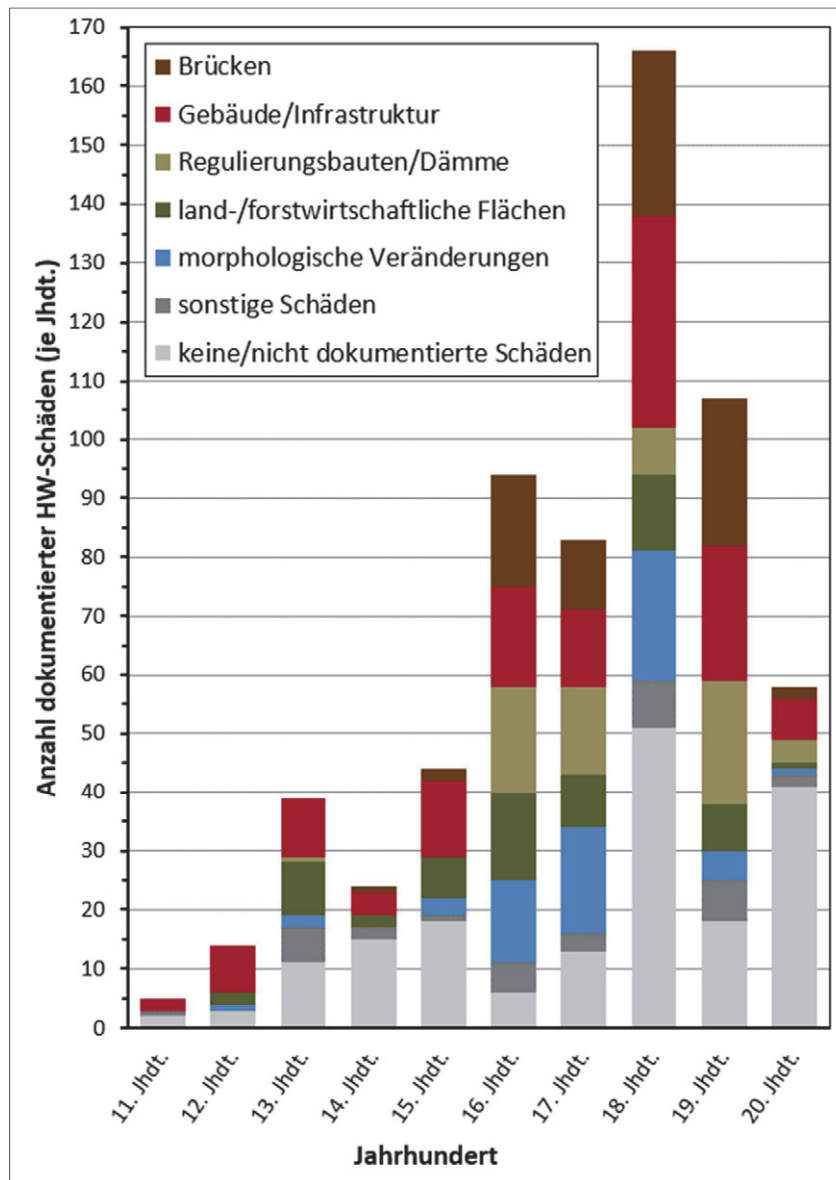
Abb. 7: Historisch dokumentierte Hochwasserschäden an der Wiener Donau seit dem 11. Jahrhundert.
