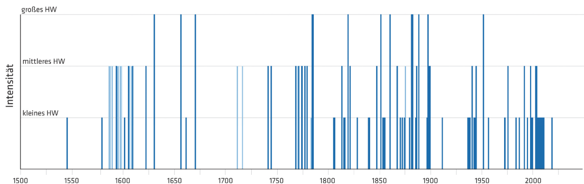
Abb. 8: Historisch dokumentierte Hochwässer am Wienfluss im heutigen Wiener Stadtgebiet seit dem Jahr 1500. Für den Zeitraum vor 1500 sind größere Hochwässer lediglich für die Jahre 1221, 1295, 1405 und 1445 verzeichnet (hellblau: Hochwässer mit schlecht dokumentierter Intensität).
