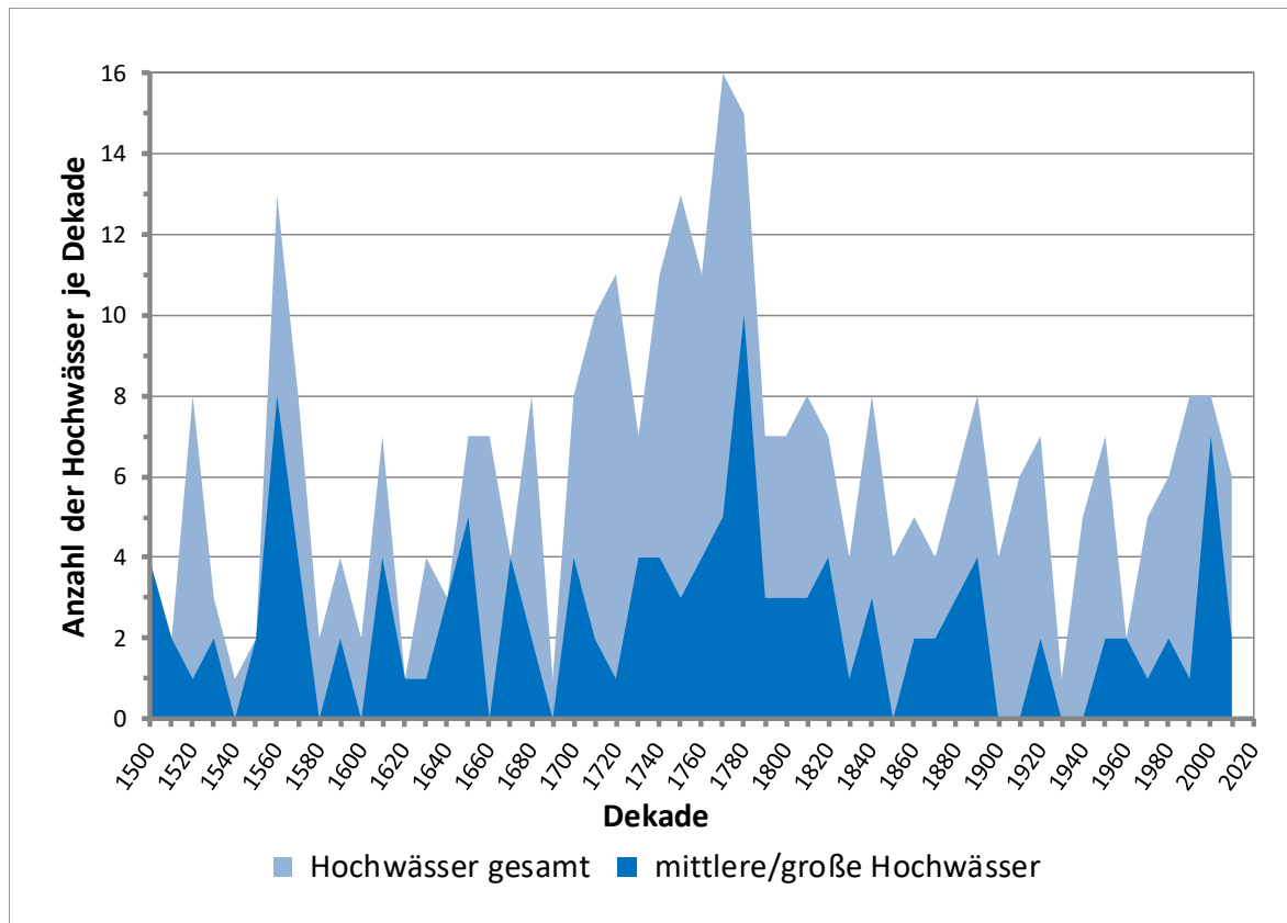
Abb. 3: Anzahl dokumentierter Hochwässer je Dekade bei Wien (Donau ohne Zubringer) seit 1500 n. Chr. In den letzten 500 Jahren sind primär drei Phasen mit verstärkter Hochwasseraktivität bemerkbar: ein erster Anstieg in den 1560ern, eine zweite, noch intensivere Phase im 18. Jahrhundert, und zuletzt seit Ende des 20. Jahrhunderts.
