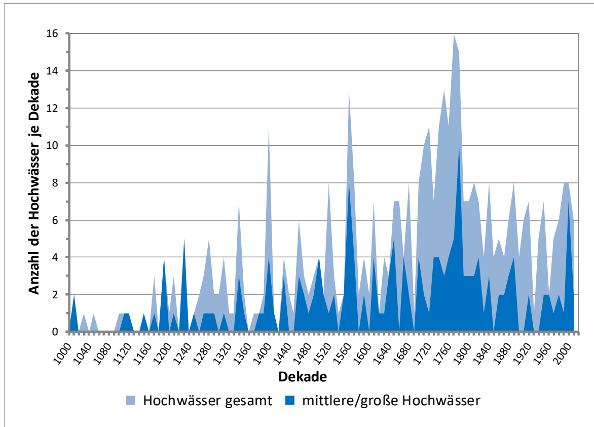
Abb. 2: Anzahl der historisch dokumentierten Hochwässer je Dekade bei Wien (Donau ohne Zubringer) seit 1000 n. Chr. (vor 1500 n. Chr. liegen nur fragmentarische Informationen vor).
